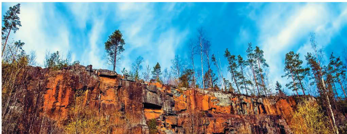
Памятник природы «Щелейки» расположен в Подпорожском районе, на юго-западном побережье Онежского озера. Здесь на поверхность выходят скальные породы южной оконечности Шокинской гряды, образованной кварцито-песчаниками, кварцитами, диабазами и габбро-диабазами. Скалы поднимаются на высоту до 100 м над уровнем озера.
